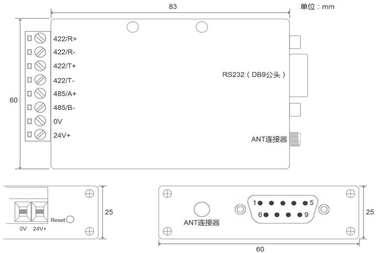
图 3.1 LORA 模块尺寸图
